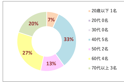
(2) 年代
